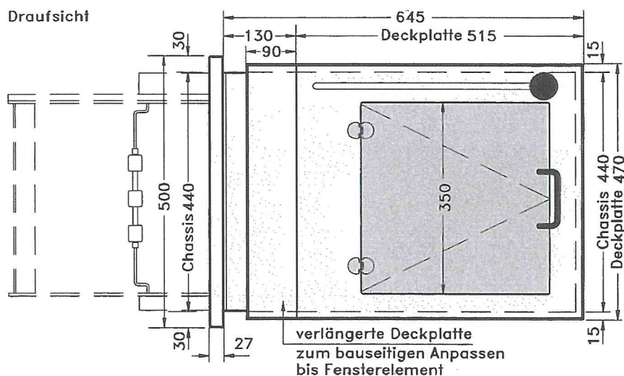
Draufsicht
